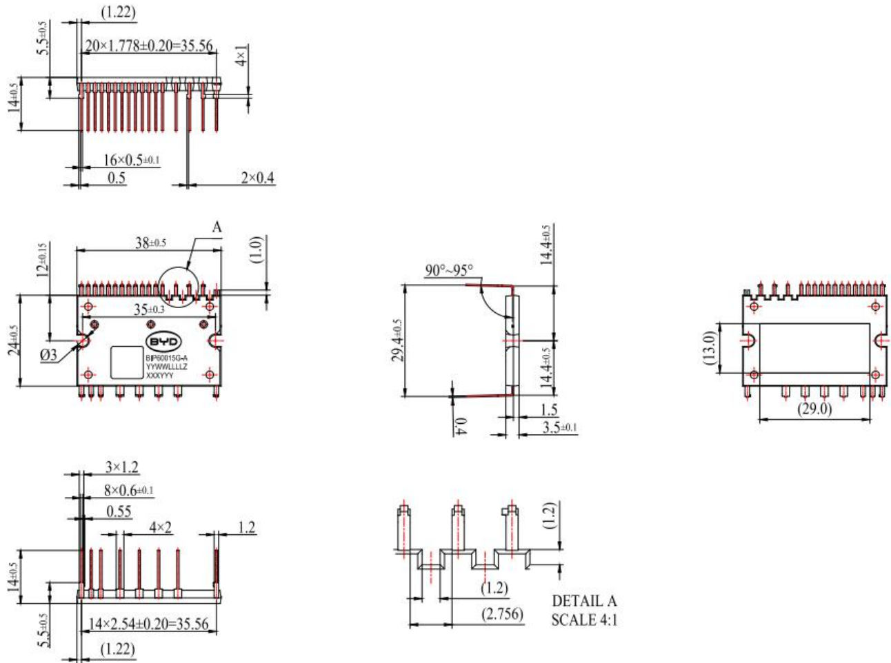
图 9. 封装轮廓详图
