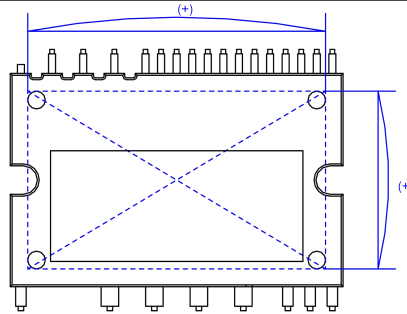
图 5. 平面度测量位置 Fig 5. Flatness Measurement Position
