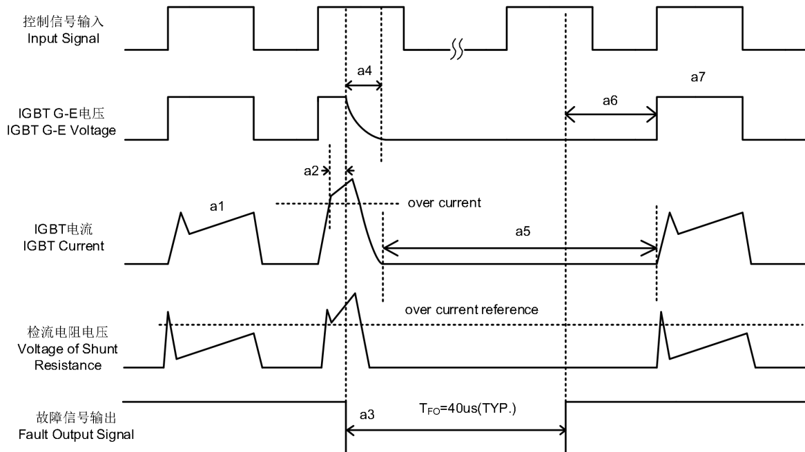
图 6.过流保护
