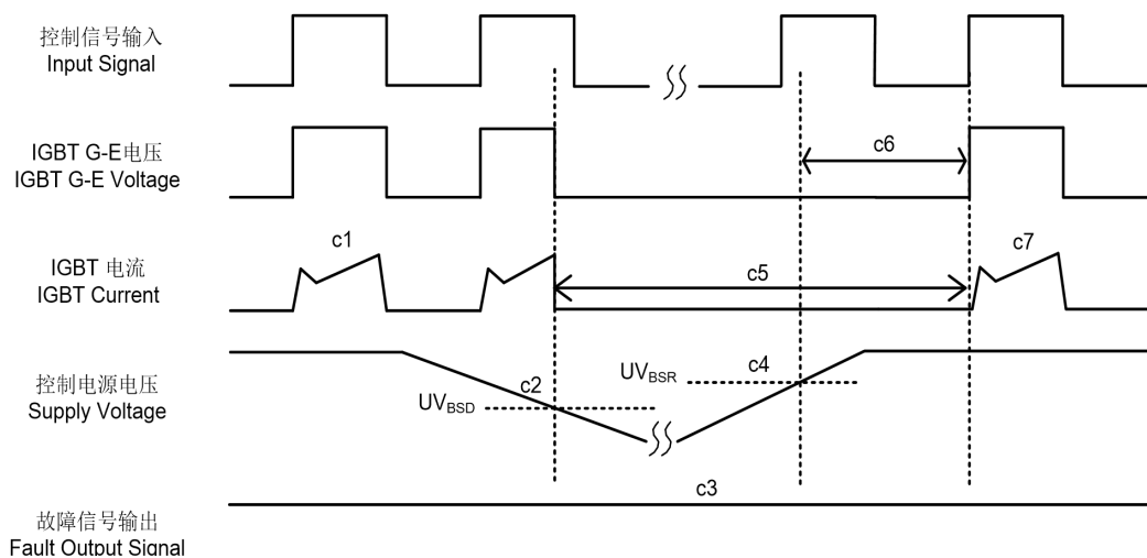
图 8. 上桥欠压保护
